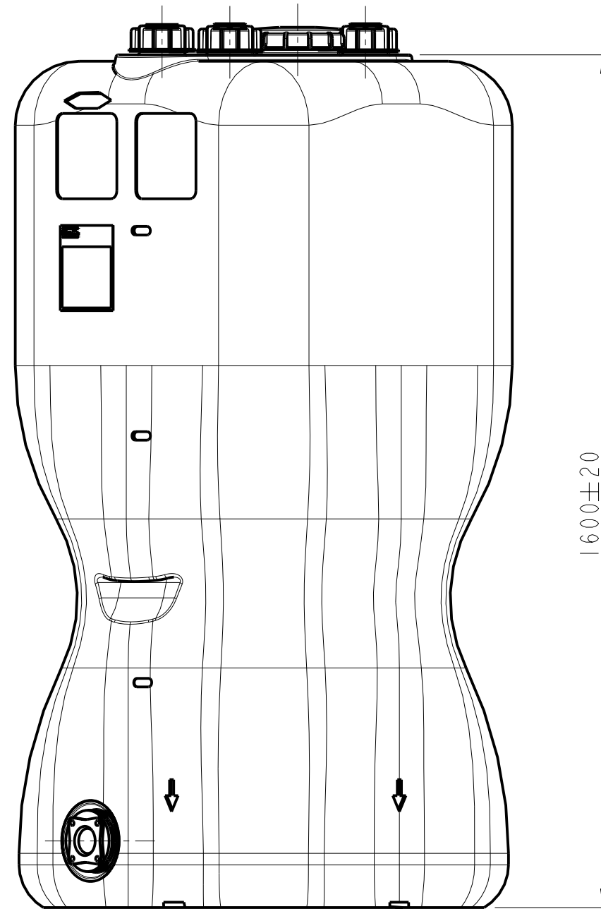
Widok A
